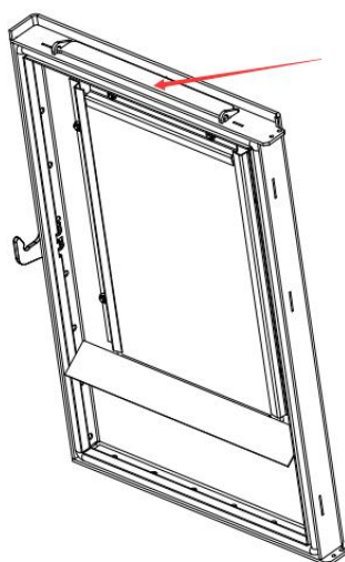
Proti-explozivní klapka
