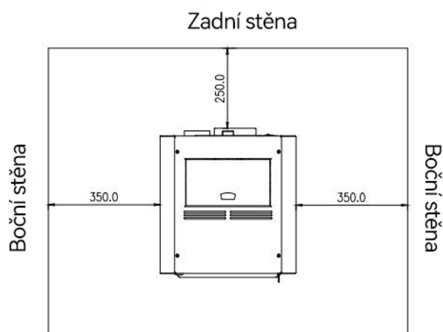
Paralelní instalace
