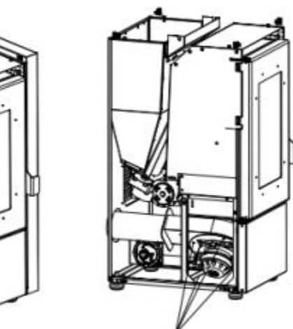
Odpojte kabely od odsávacího ventilátoru, imbusovým klíčem 4 mm odšroubujte upevňovací šrouby a vyjměte jednotku k vyčištění.
